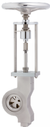
Segmentplattenventil mit Handantrieb 5050 Nennweite: DN 25 - 200 Nenndruck: PN 25 Werkstoff: Edelstahl (ab DN 150 auch in C-Stahl) Antrieb: Leichtgängiger kugel- gelagerter Handantrieb
