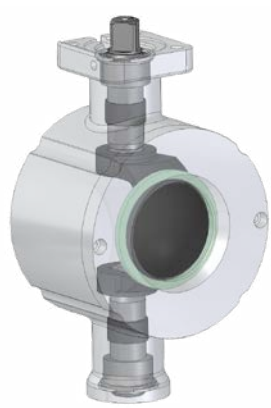
Standard Drehkegelventil geschlossen
